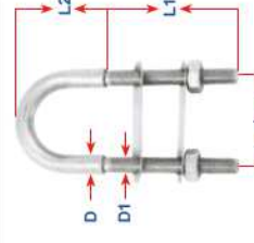
Art. n° 8230 Cavallotto ad “U” “U” bolt
