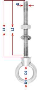
Art. n° 8267 Bullone con occhio Eye bolt
