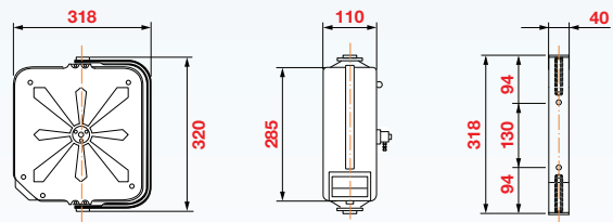
DIMENSIONI D'INGOMBRO
